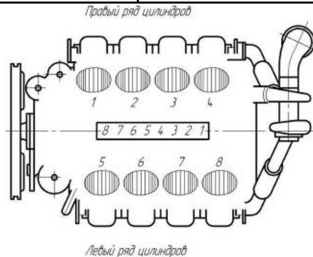
Схема нумерации цилиндров и секций ТНВД
