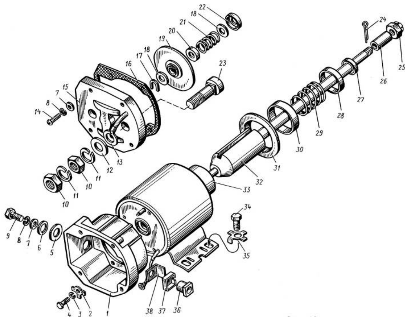
Рис.39 Реле стартера
