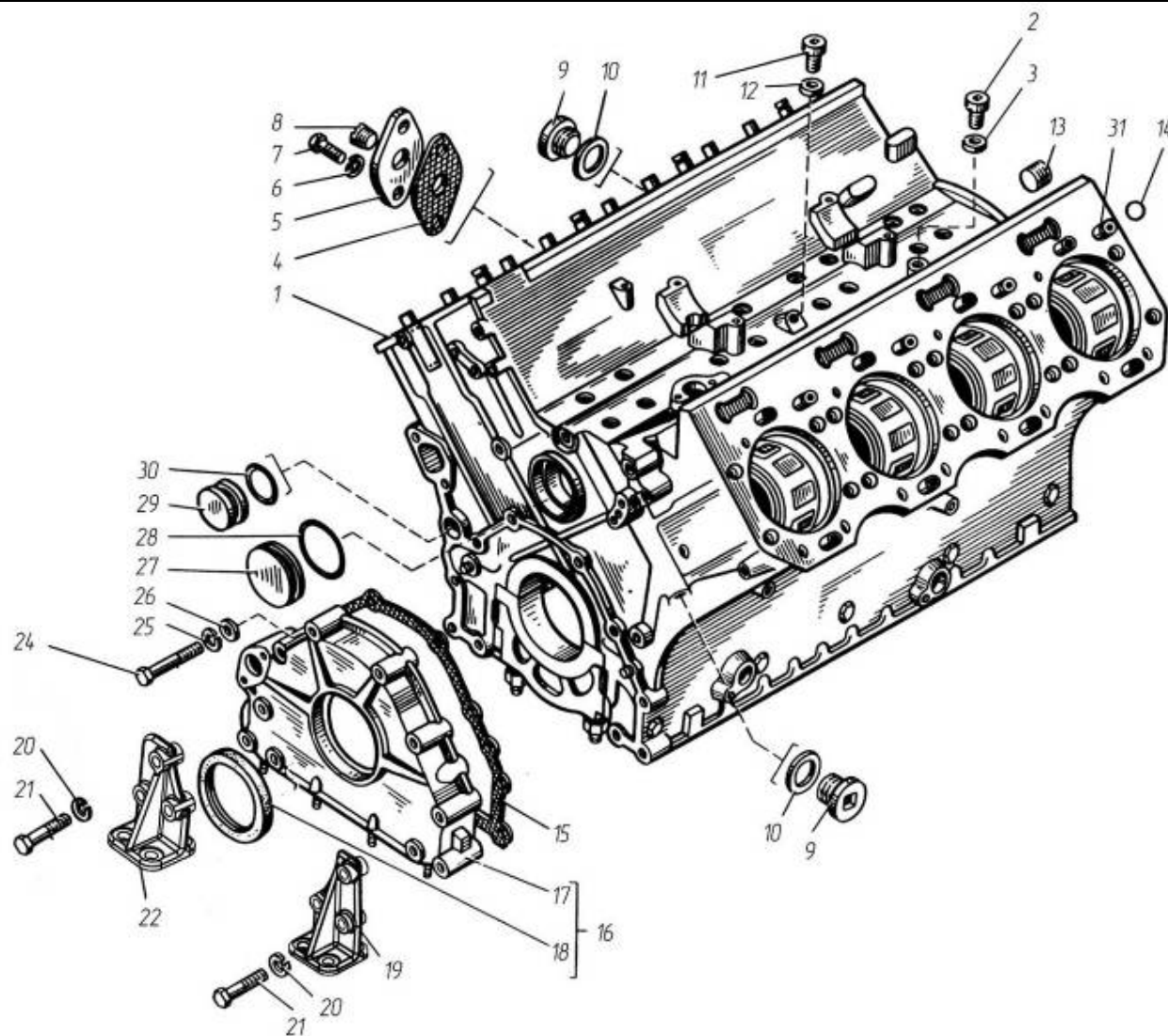
Рис.1 Блок цилиндров и передняя опора
