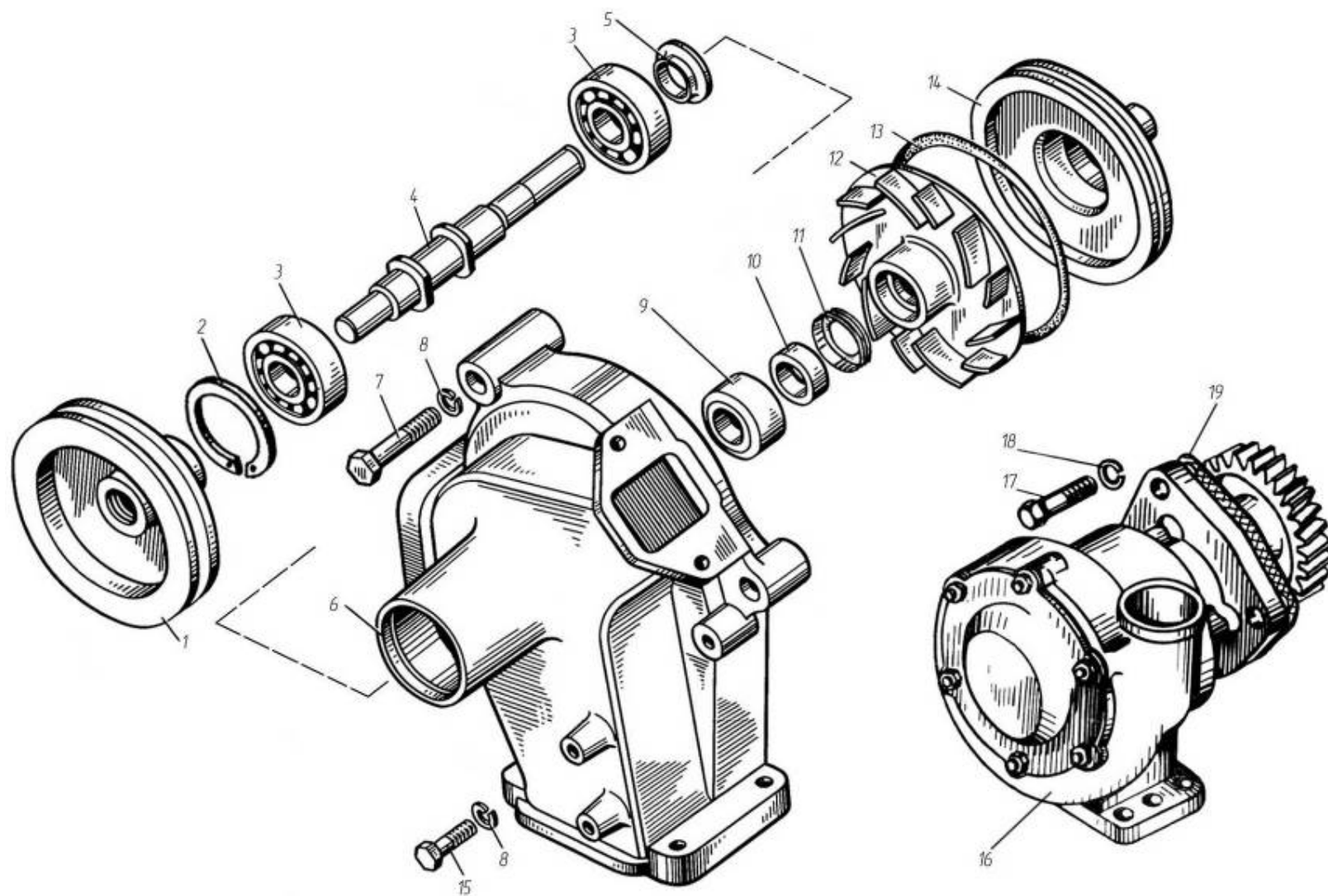
Рис.32 Водяной насос
