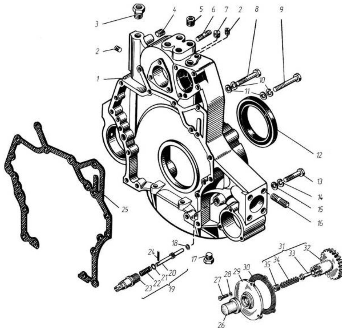
Рис.2 Картер маховика
