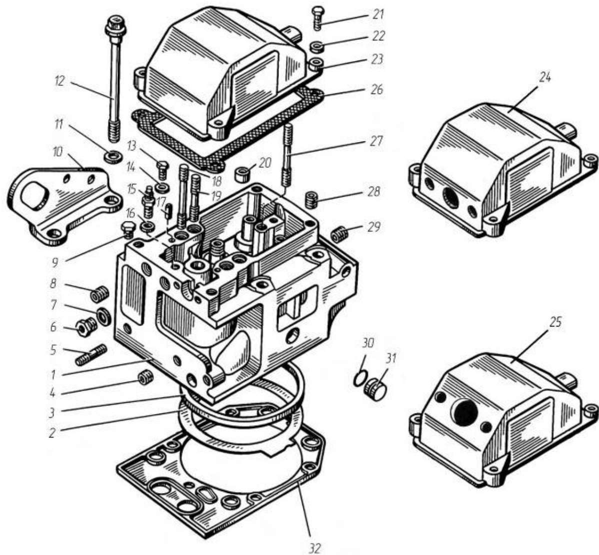
Рис. 3 Головка цилиндра
