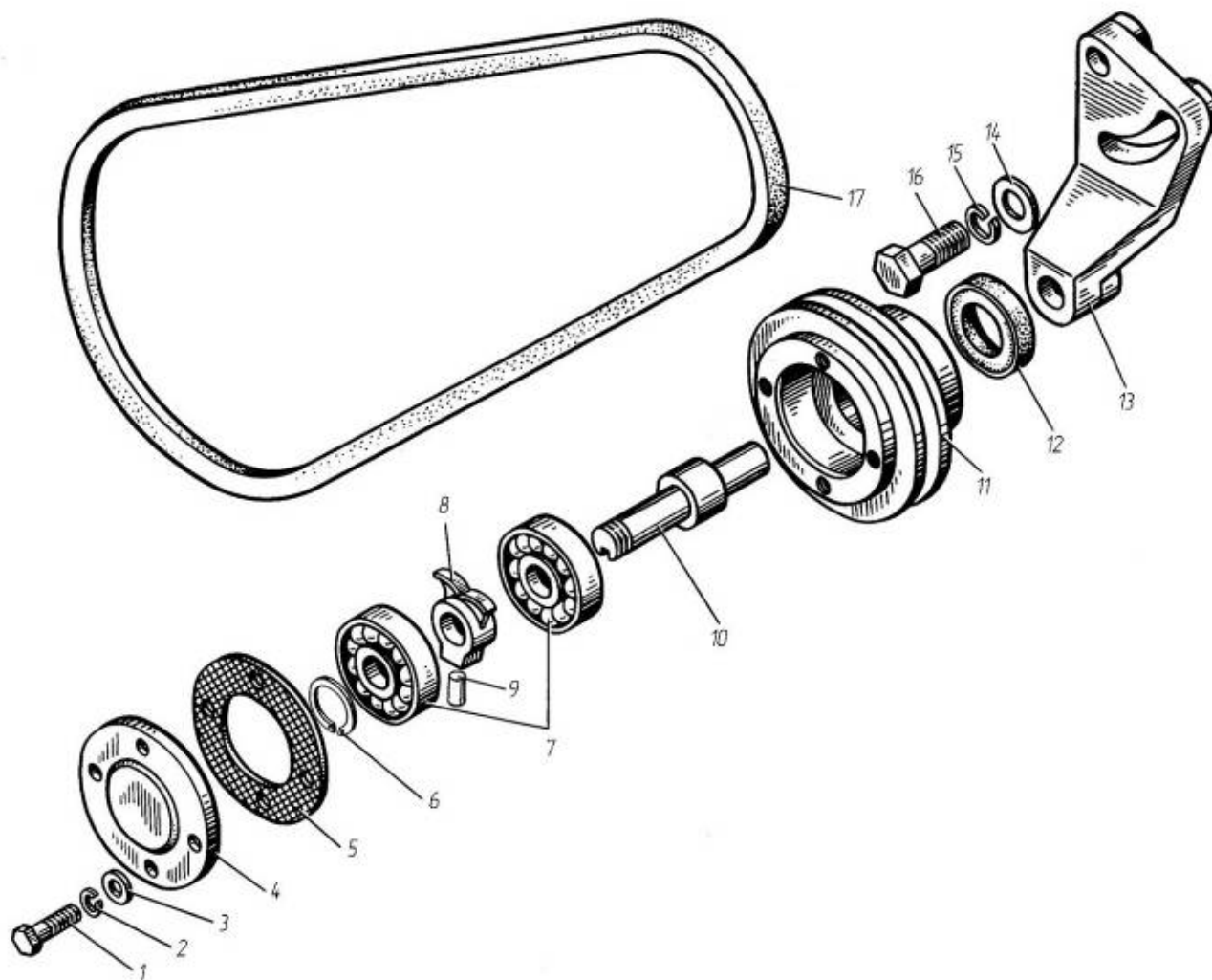
Рис.33 Натяжное устройство
