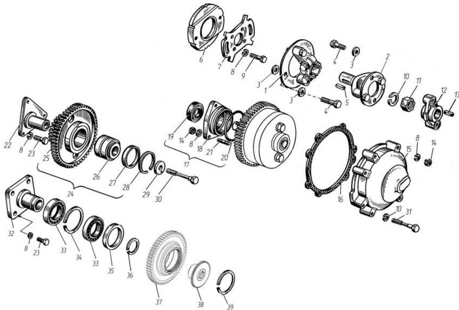
Рис.16 Привод агрегатов
