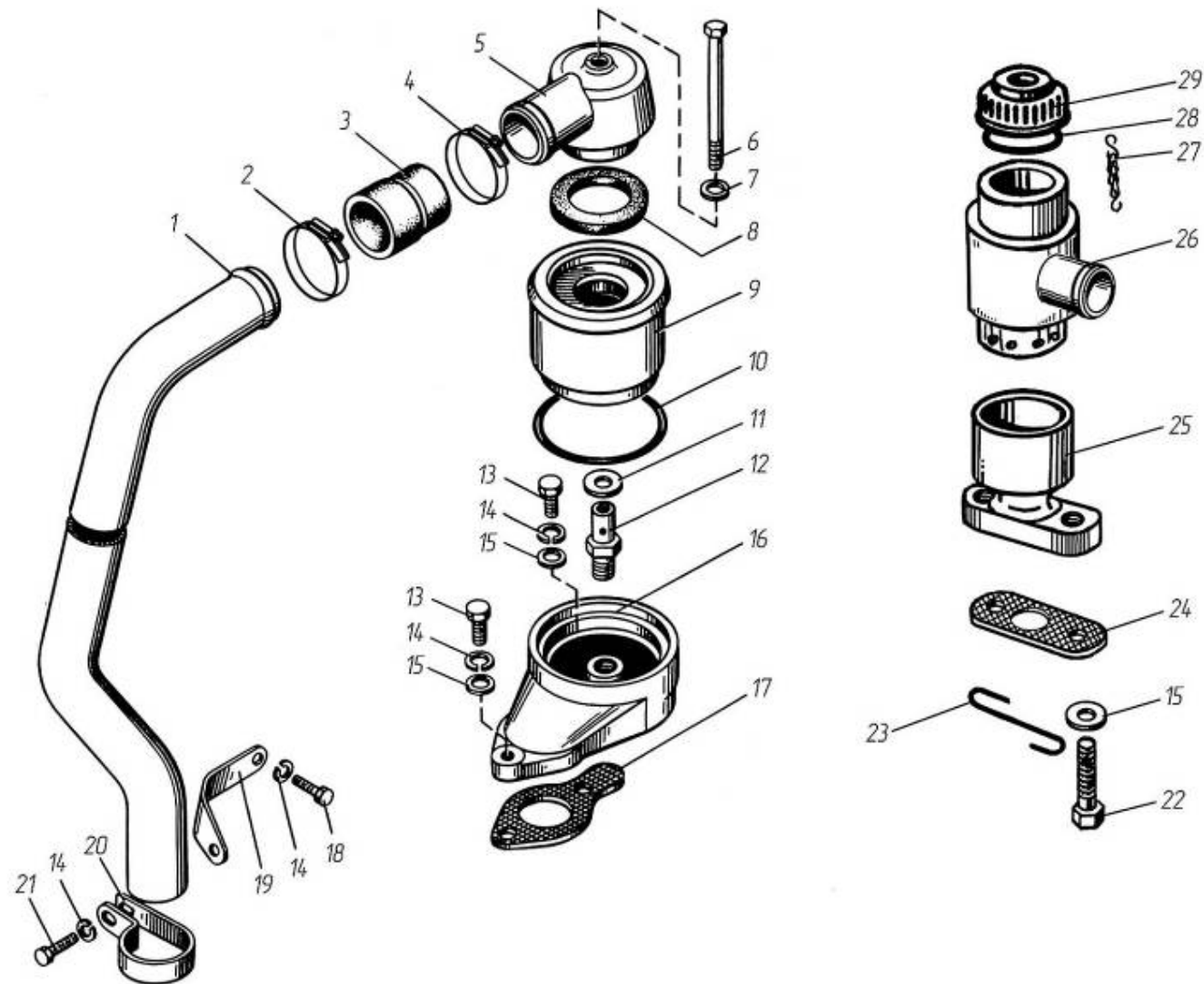
Рис.13 Вентиляция картера
