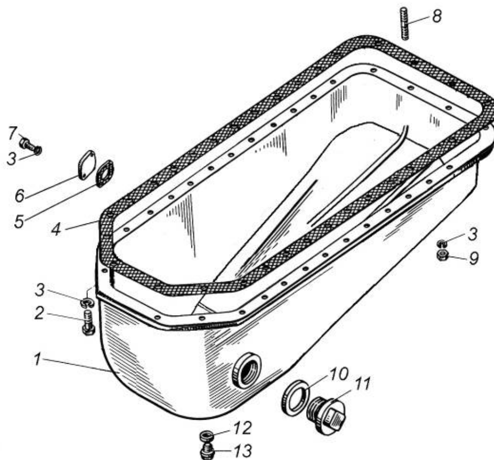
Рис. 9 Картер масляный (поддон)
