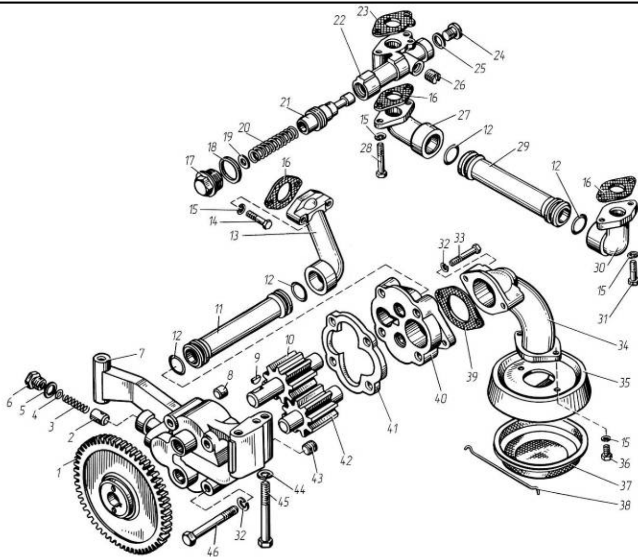
Рис. 10 Насос масляный
