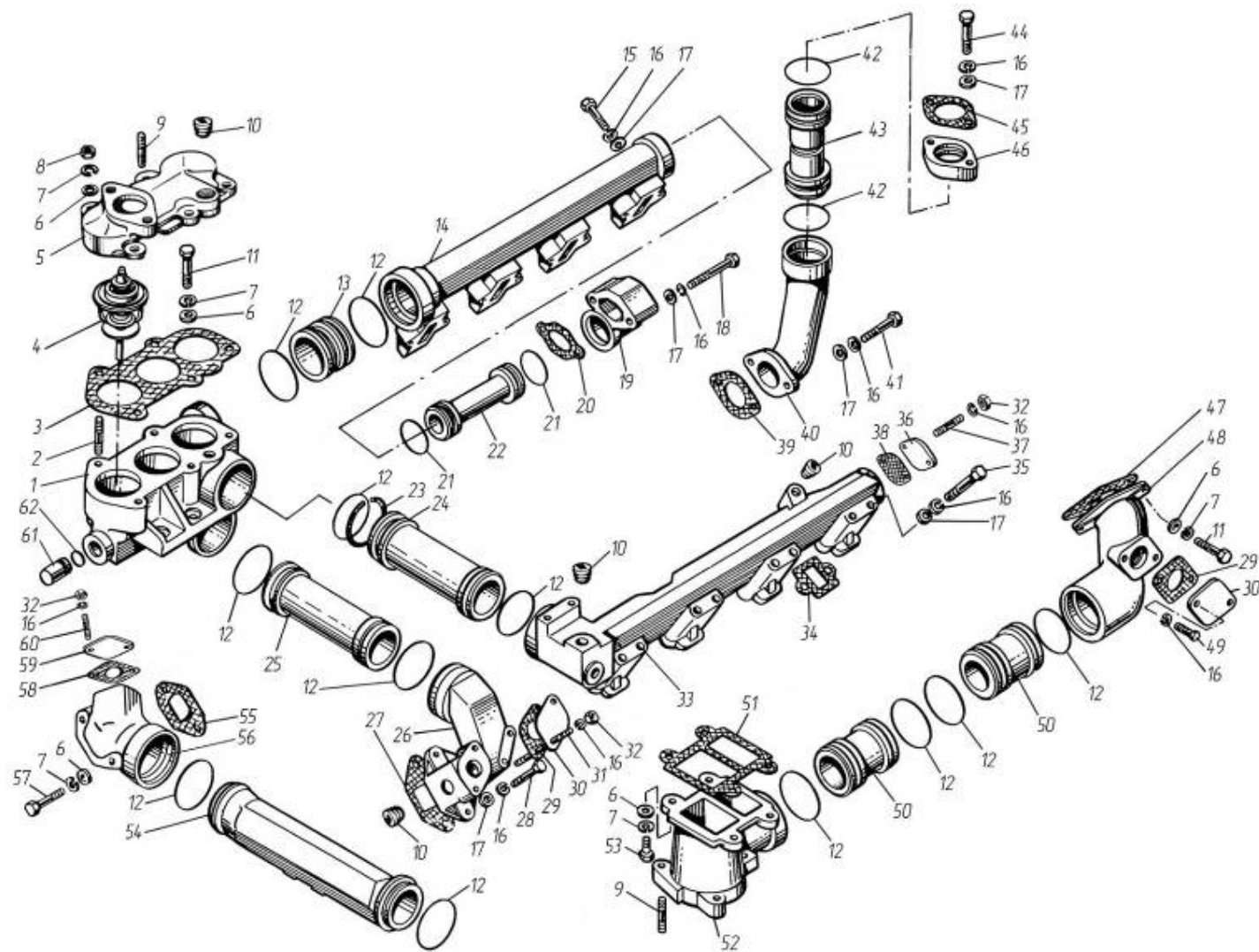
Рис.31 Трубы и термостаты системы охлаждения
