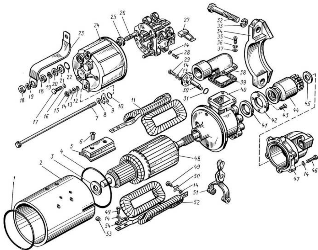
Рис.38 Стартер
