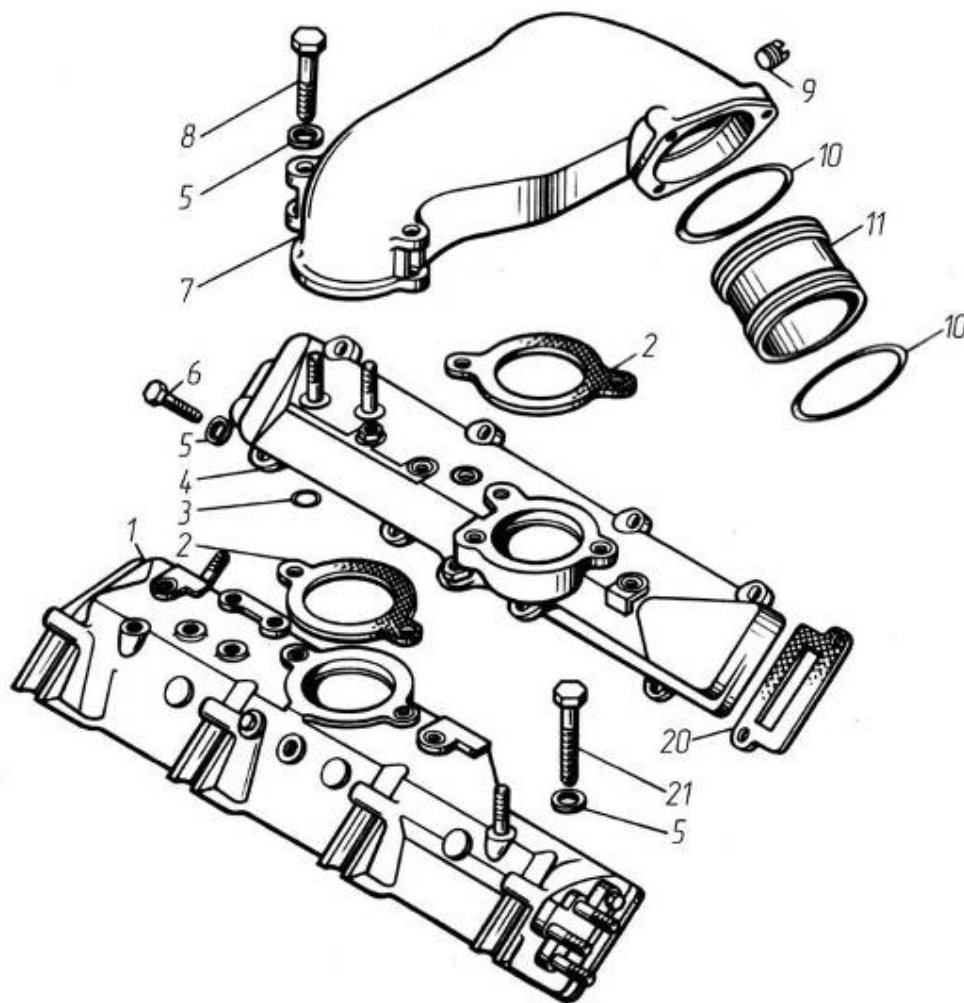
Рис.26 Впускные коллекторы
