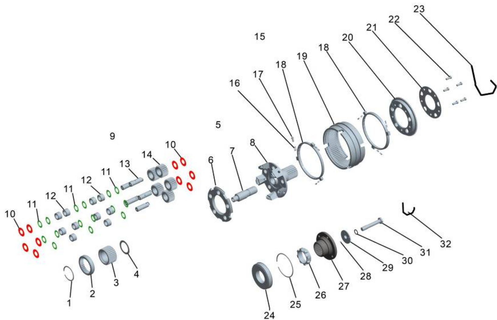
Рис.10 Вал и шестерни демультипликатора коробки передач.
