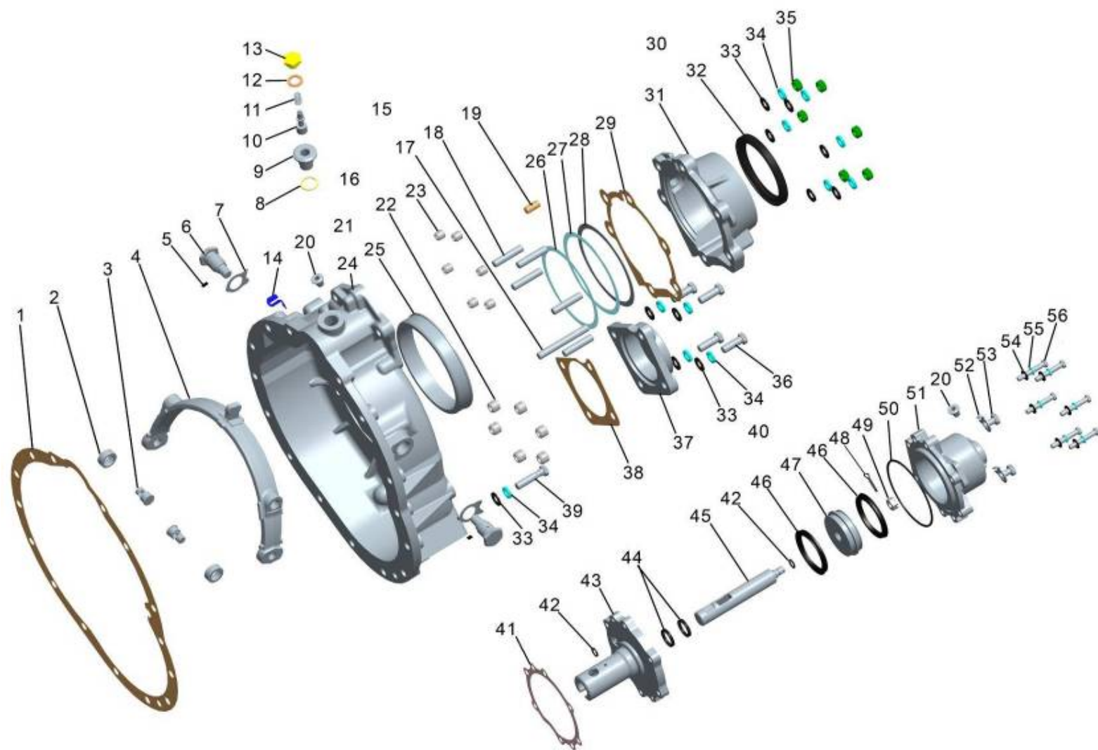
Рис.11 Картер демультипликатора коробки передач.
