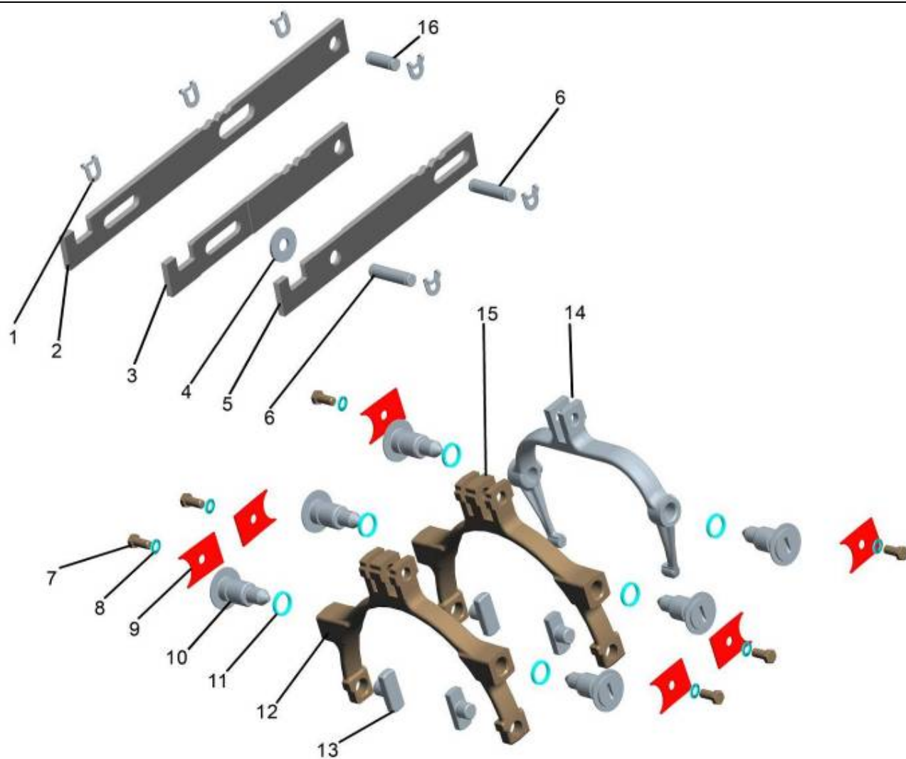
Рис. 7 Механизм переключения передач.
