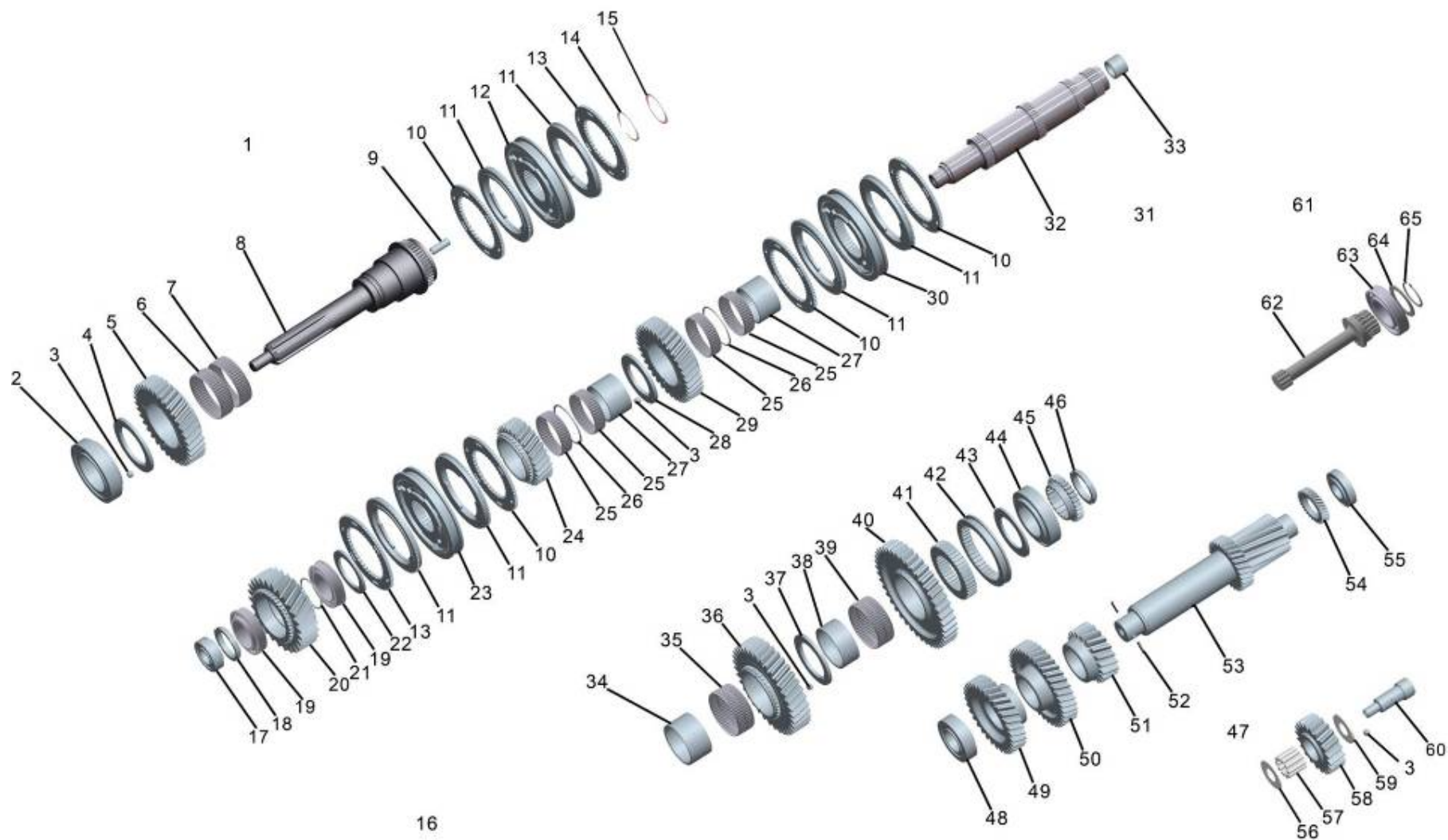
Рис. 6 Валы и шестерни коробки передач.
