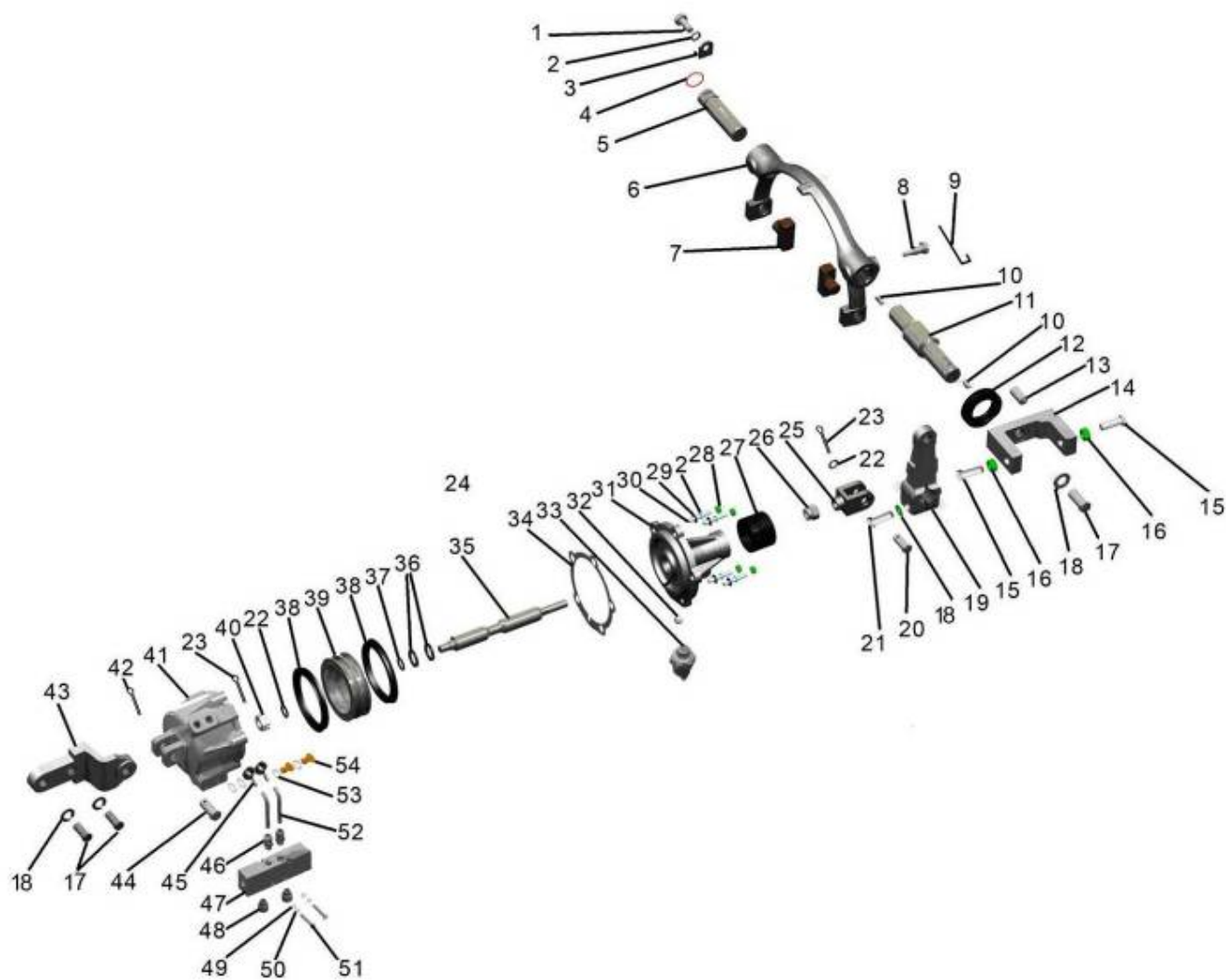
Рис. 9 Механизм переключения делителя.
